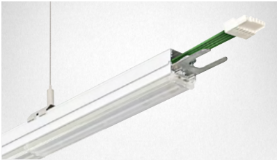
Anfangs-/Mitteelement mit LED Linear Modulen, Einspeisung und Durchgangs-verdrahtung
